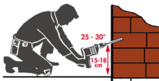
MISURE SPEEDY DIAM. 32MM, L. 30CM (POSSIBILE ACCORCIARLA)
