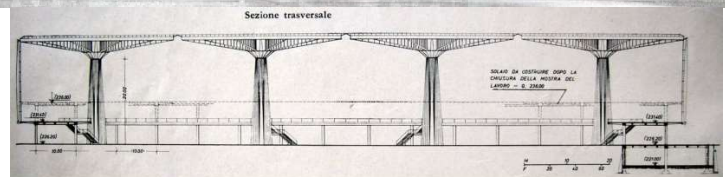
SEZIONI PROSPETTICHE DEL PALAZZO DEL LAVORO REALIZZATE DALLO STUDIO NERVI BARTOLI NELL'OTTOBRE 1959
